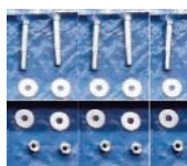
N°5 VIS M12X90 TETF ZN N.N°10 RONDELLE M12X36 H2,5 ZN N°5 ÉCROU DE SÉC. M12 ZN
